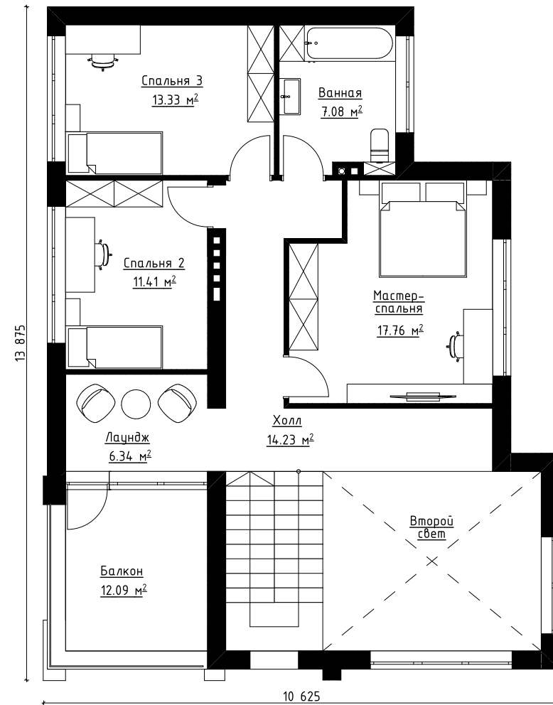
2-й этаж
