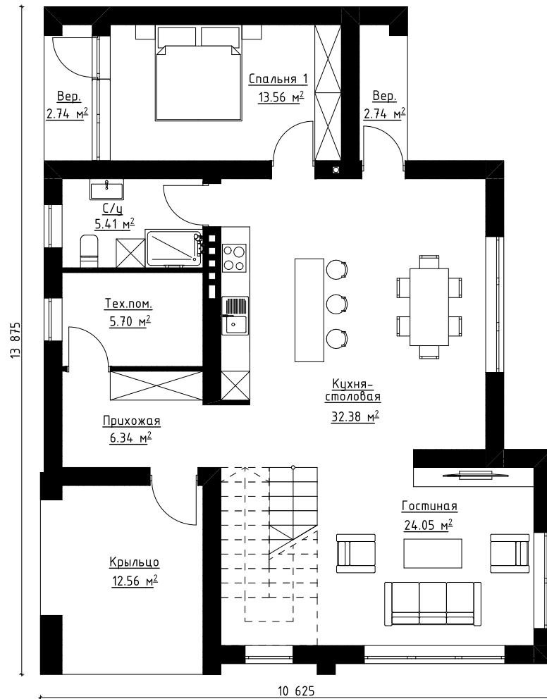
1-й этаж
